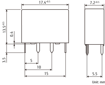
FTR-P3CN***W1 dimensions
